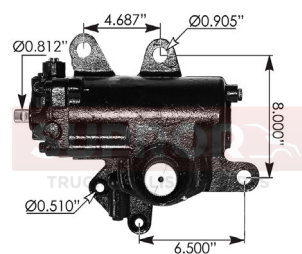
CAJA DIRECCIÓN
