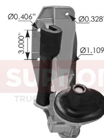
GUÍA COFRE COMPLETA R
